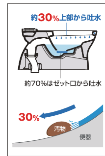
従来型ゼット口付便器
